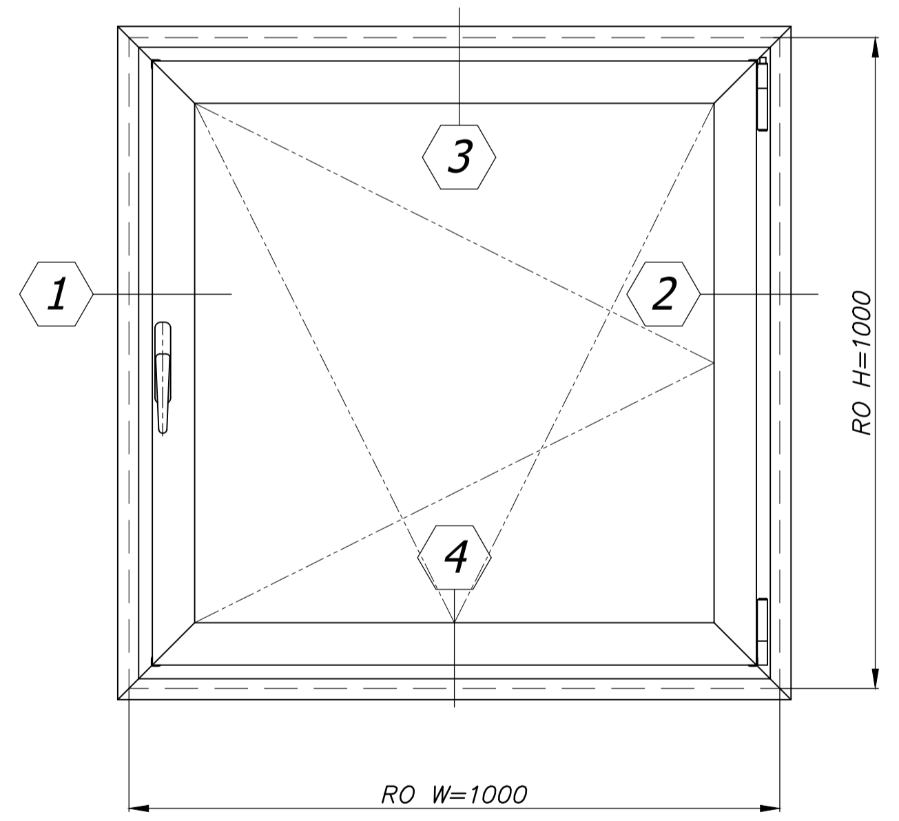
מבט פנים Scale 1:10
