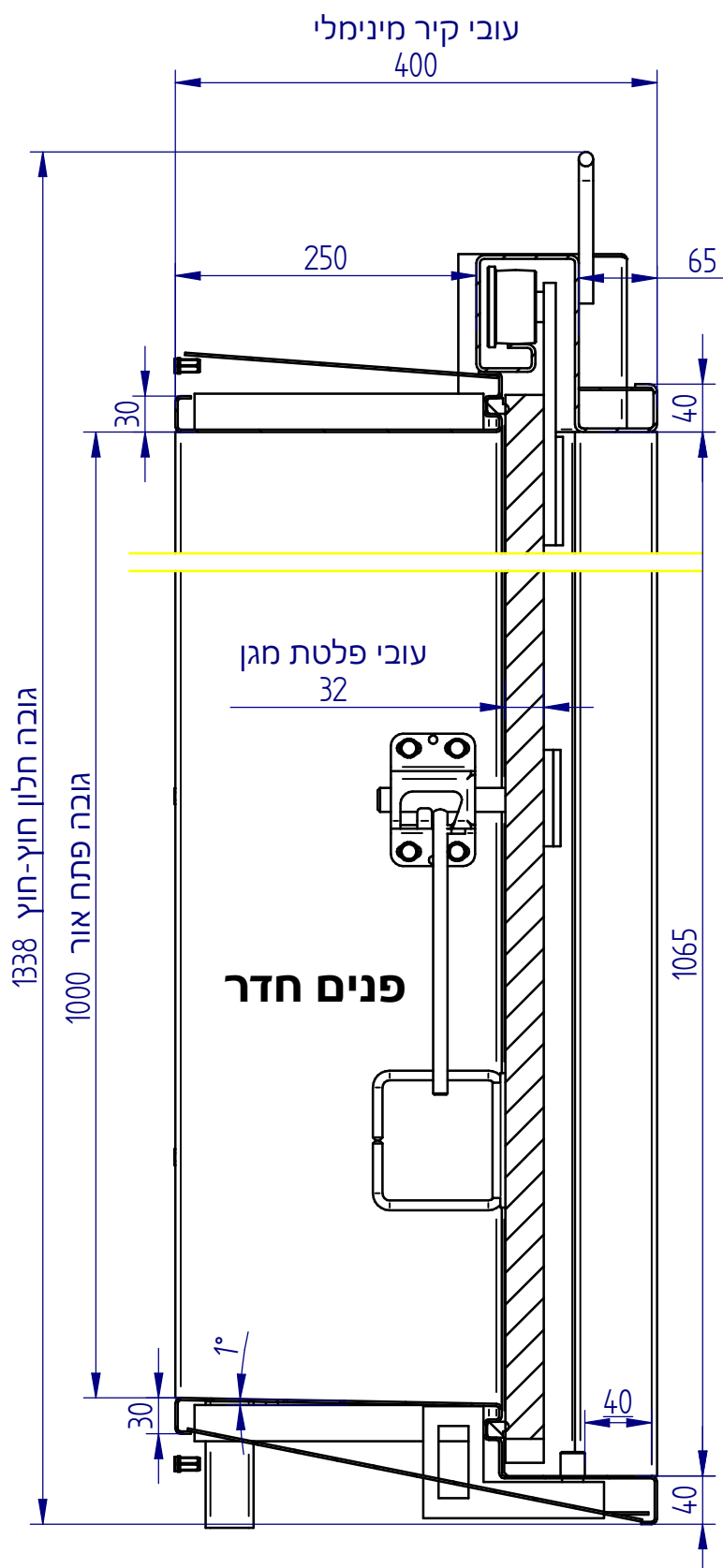
SECTION A-A
