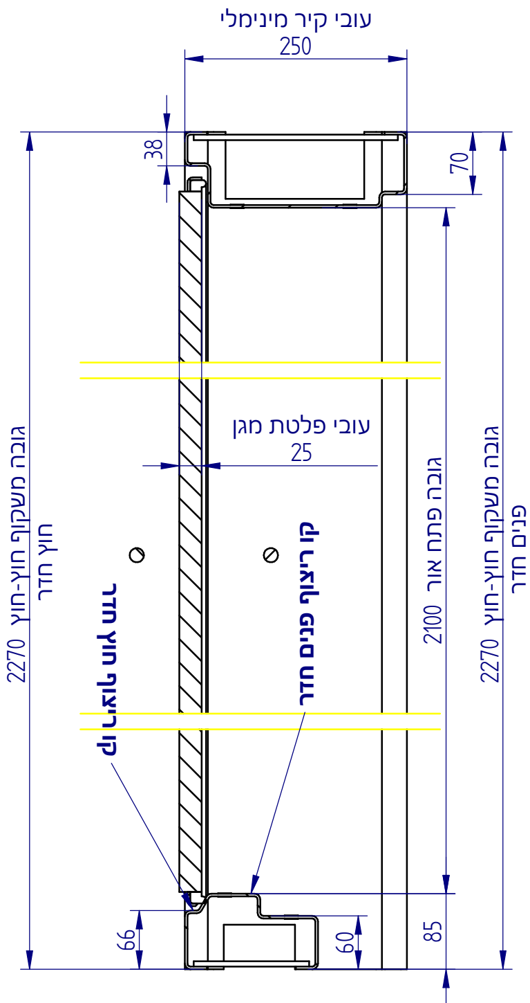
SECTION A-A
