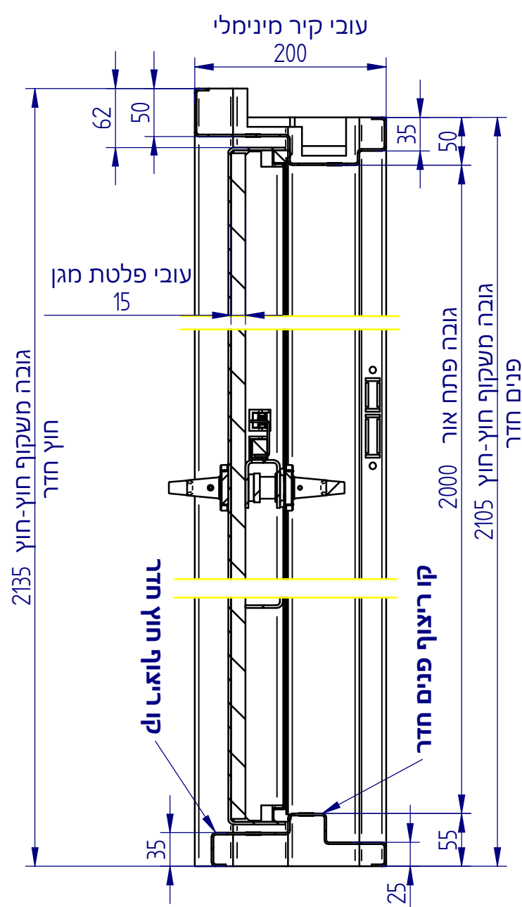
SECTION A-A
